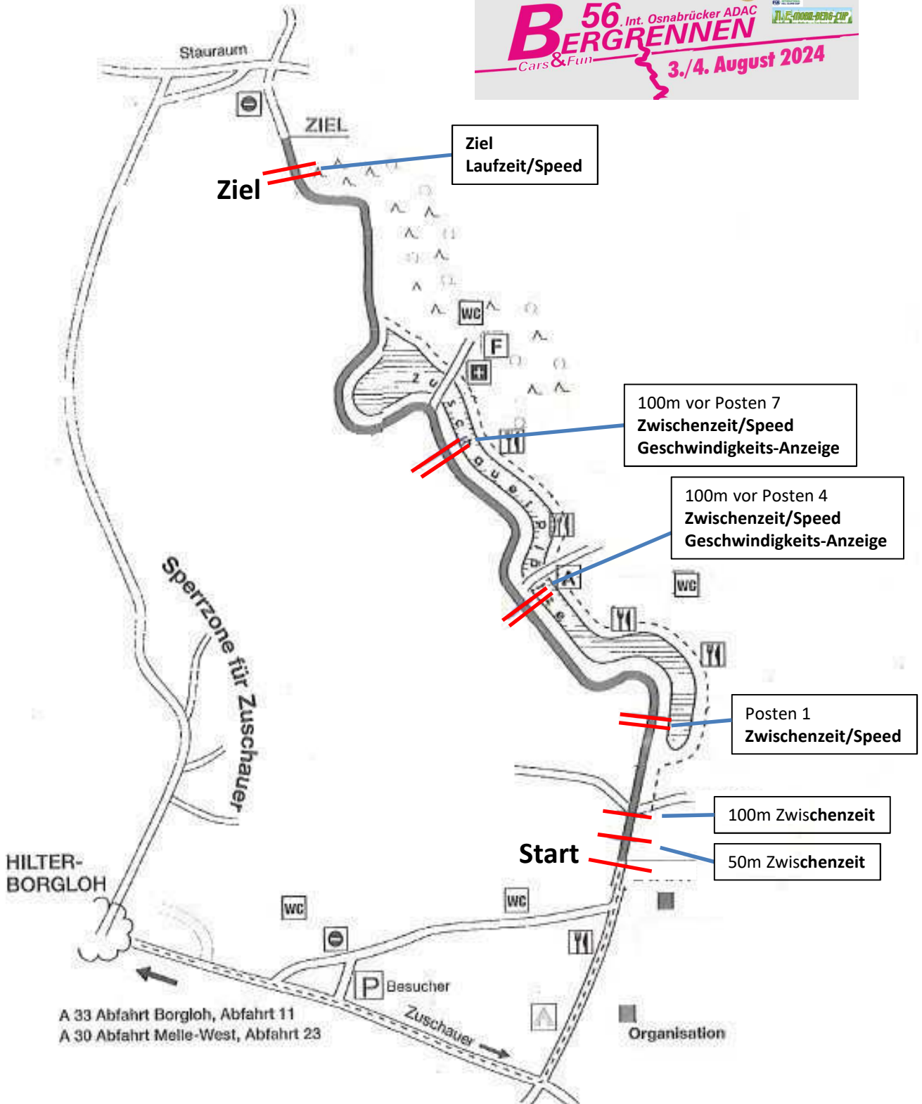
Sektorlayout/Zwischenzeiten
